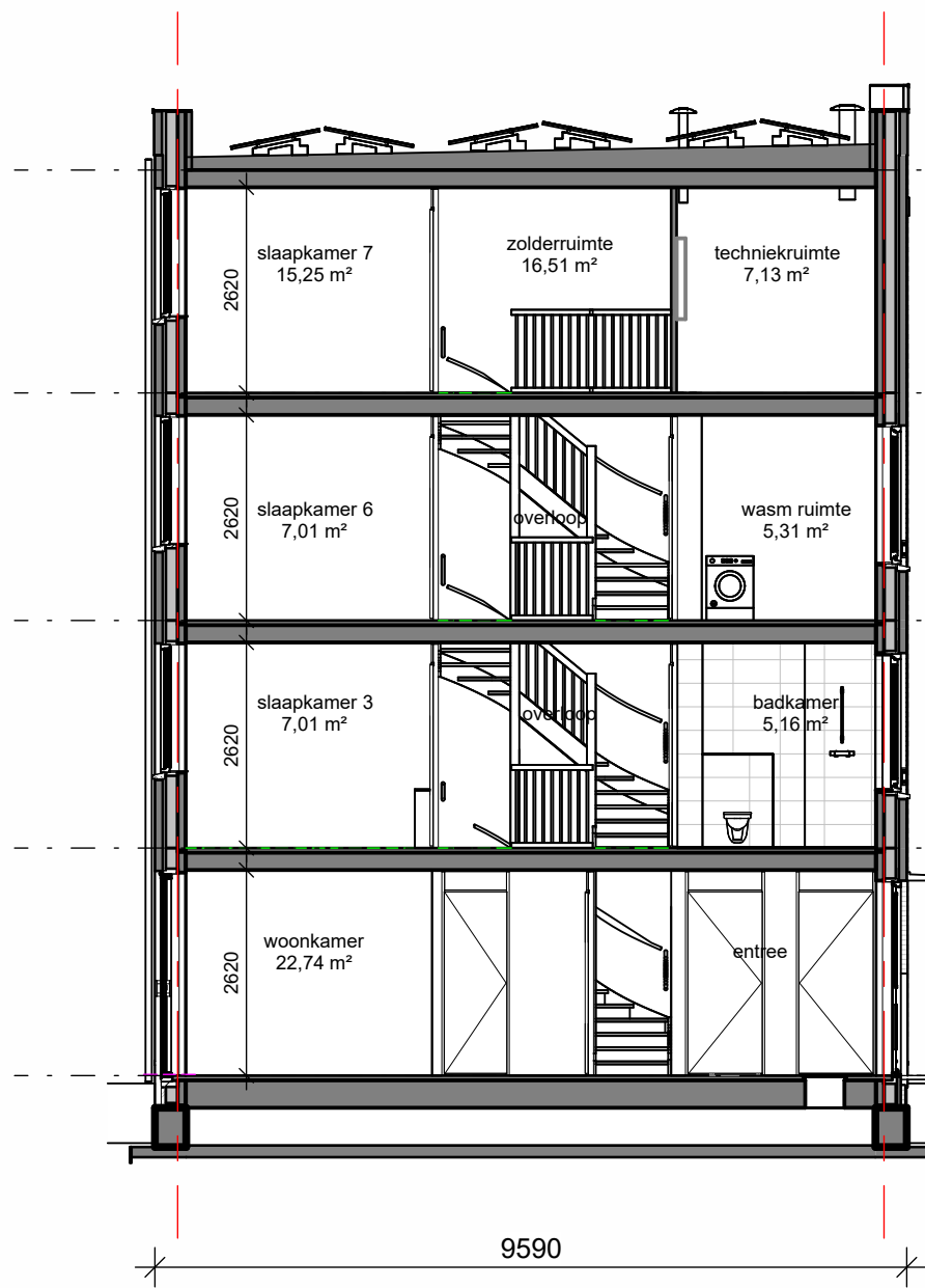
doorsnede 3b-01
