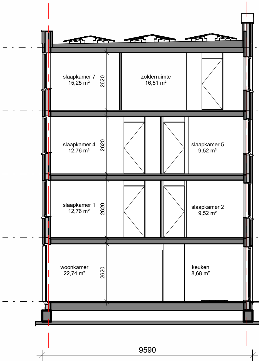
doorsnede 3b-2
